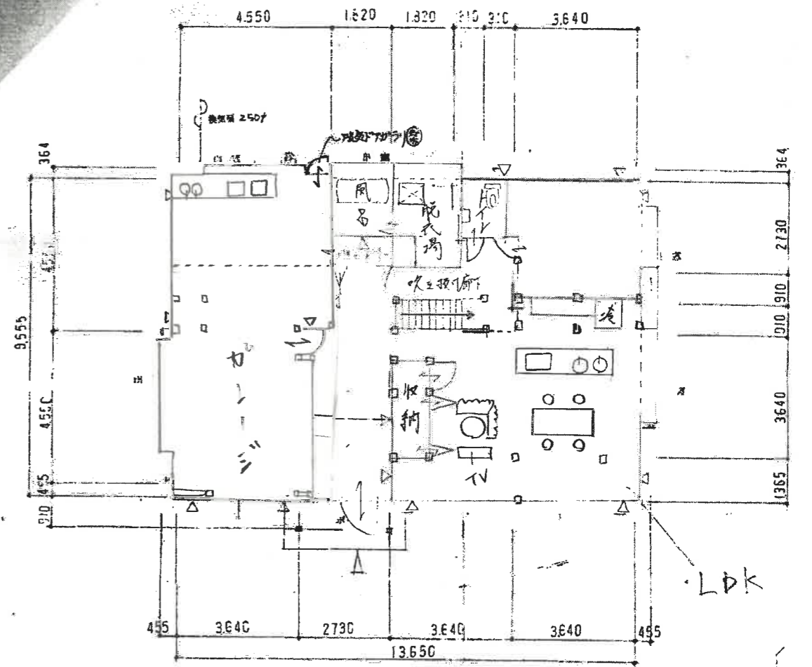
1 型 平面 図 S=1:100
